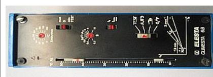
Heizungsregler ELESTA Climesta 6b
